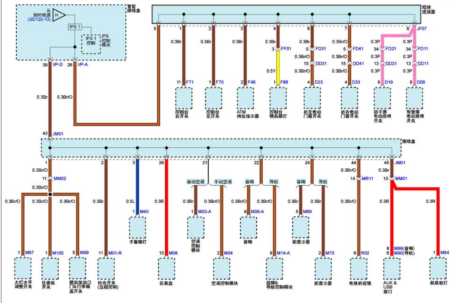
室内保险丝分布 (14)
